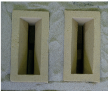
Fig. 1. Mold: a) before liquid metal pouring; b) after liquid metal pouring
