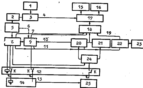
Rys. 11. Schemat blokowy urządzenia probierczego
