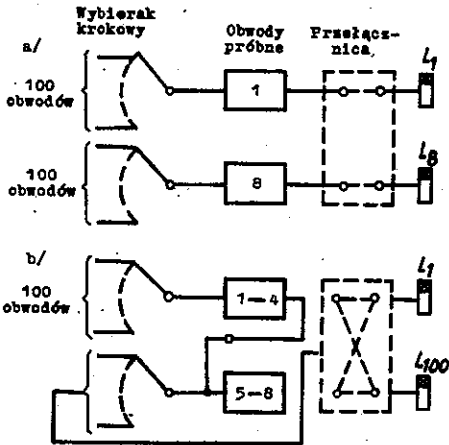
Rys. 15. Schemat blokowy urządzenia przenośnego do pomiarów ruchu telefonicznego
