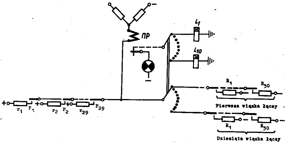
Rys. 17. Schemat ideowy miernika ruchu
