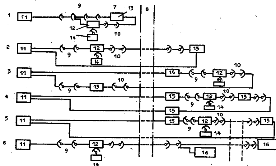
Rys. 7. Różne przypadki badań za pomocą próbnika dróg połączeniowych
