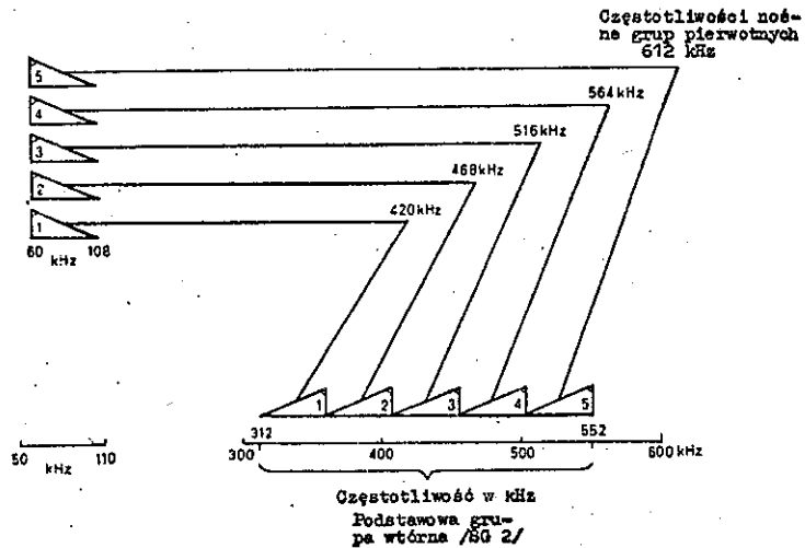
Rys. 13. Widmo podstawowej grupy wtórnej
