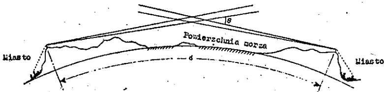
Rys. 7. Typowy przekrój trasy linii troposferycznej
