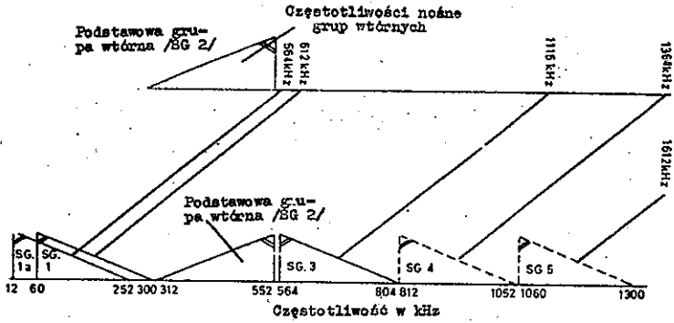
Rys. 14. Widmo grupy trójnej
