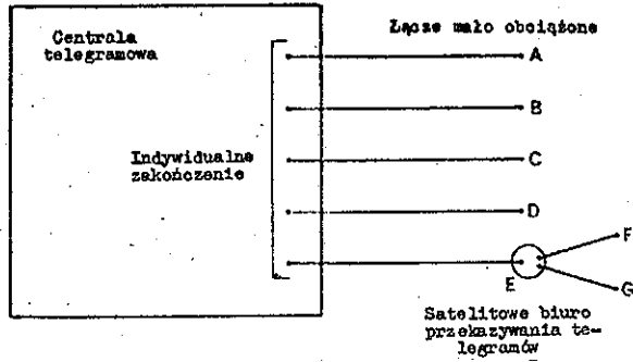
Rys. 16. Schemat blokowy przedstawiający indywidualne zakończenie w centrali telegramowej i w satelitowym biurze przekazywania telegramów w punkcie E
