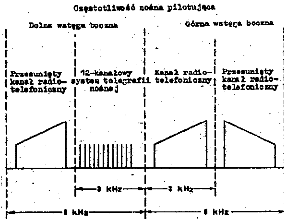
Rys. 2. Widmo częstotliwości w przypadku transmisji za pomocą niezależnych wstęg bocznych
