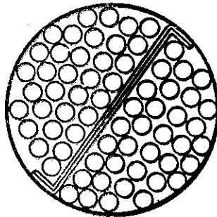
Rys. 7. Kabel o wiązkach parowych wyposażony w ekran typu Z
