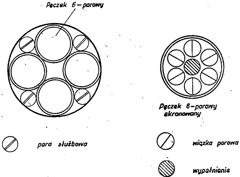
Rys. 6. Kabel 24-parowy o konstrukcji pęczkowej dla systemów PCM
