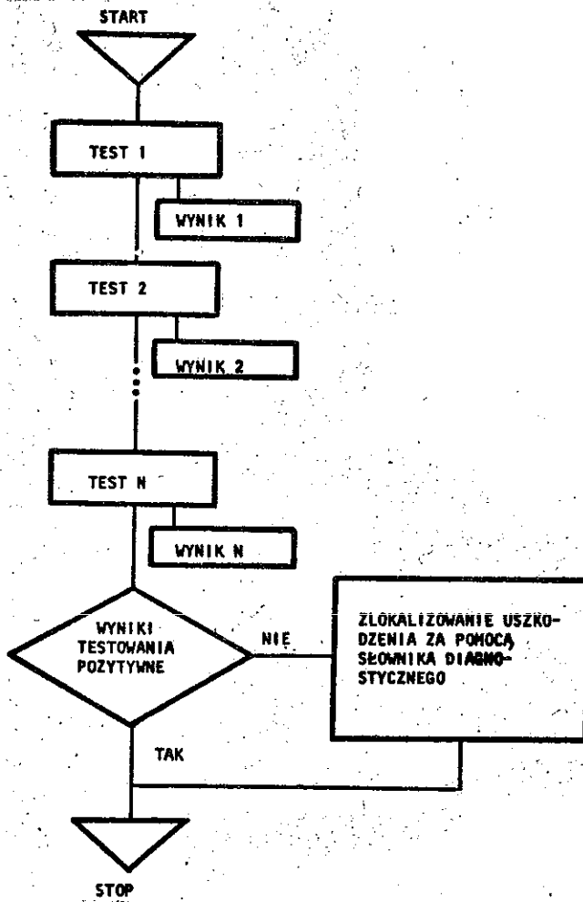
Rys. 2. Sieć działań programu diagnostycznego z procedurą kombinacyjną.
