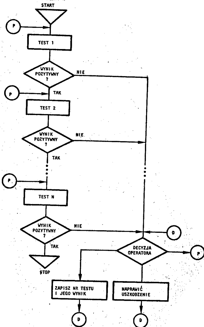
Rys. 4. Sieć działań procedury BOOTSTRAP
