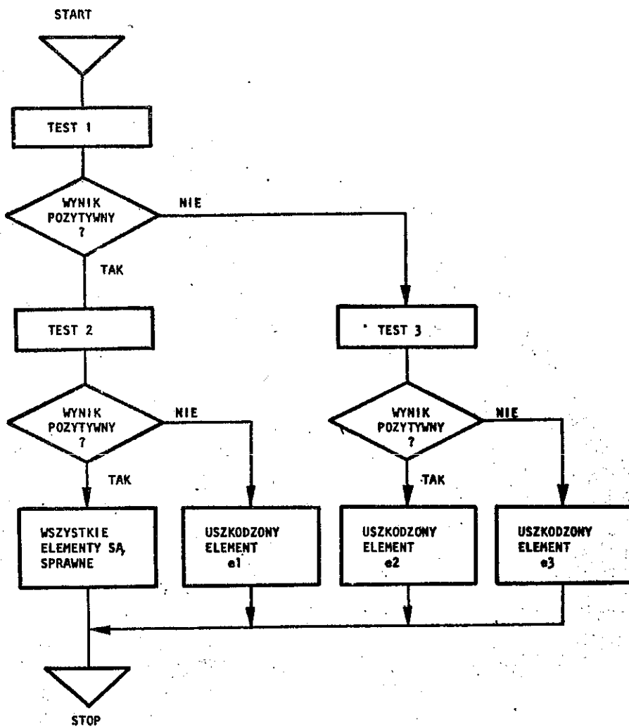
Rys. 3. Sieć działań przykładowej procedury sekwencyjnej
