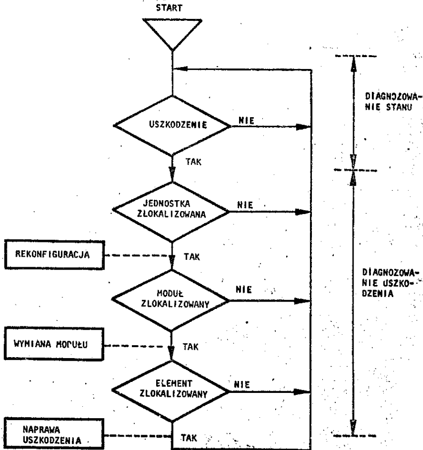
Rys. 7. Proces diagnostyczny w programowo sterowanej centrali telefonicznej
