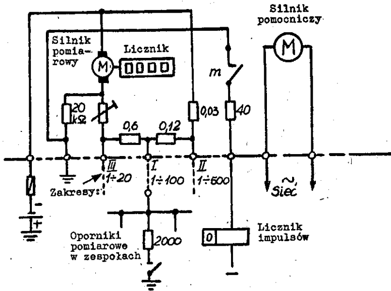
Rys. 19. Układ erlangomierza
