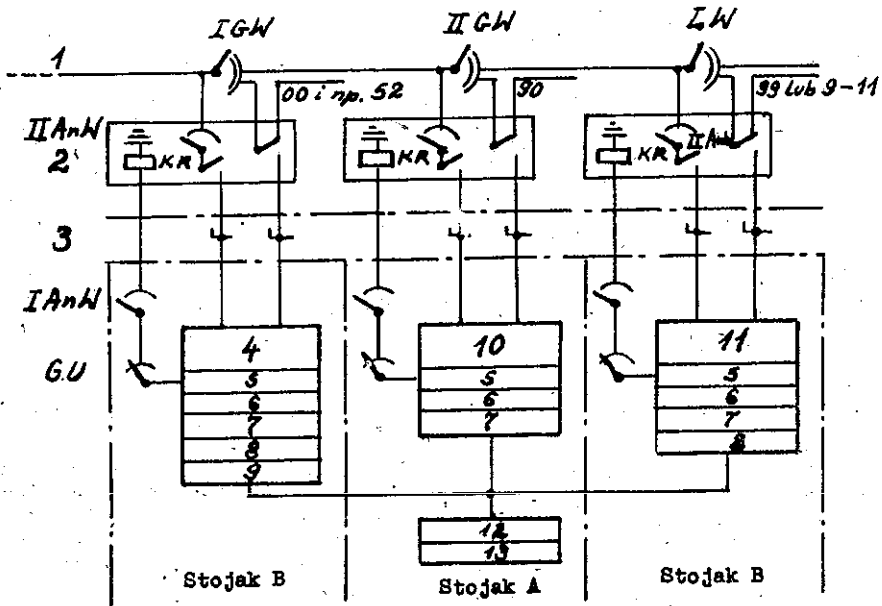
Rys. 14. Automatyczny próbnik APrE 50
