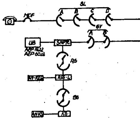
Rys. 9. Układ dołączania próbnika AEP 1622 do badanych łączy abonenckich za pomocą zespołu SNPR
