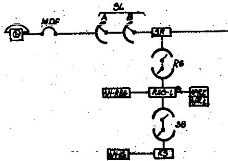
Rys. 10. Układ wybierania robota próbierczego APR
