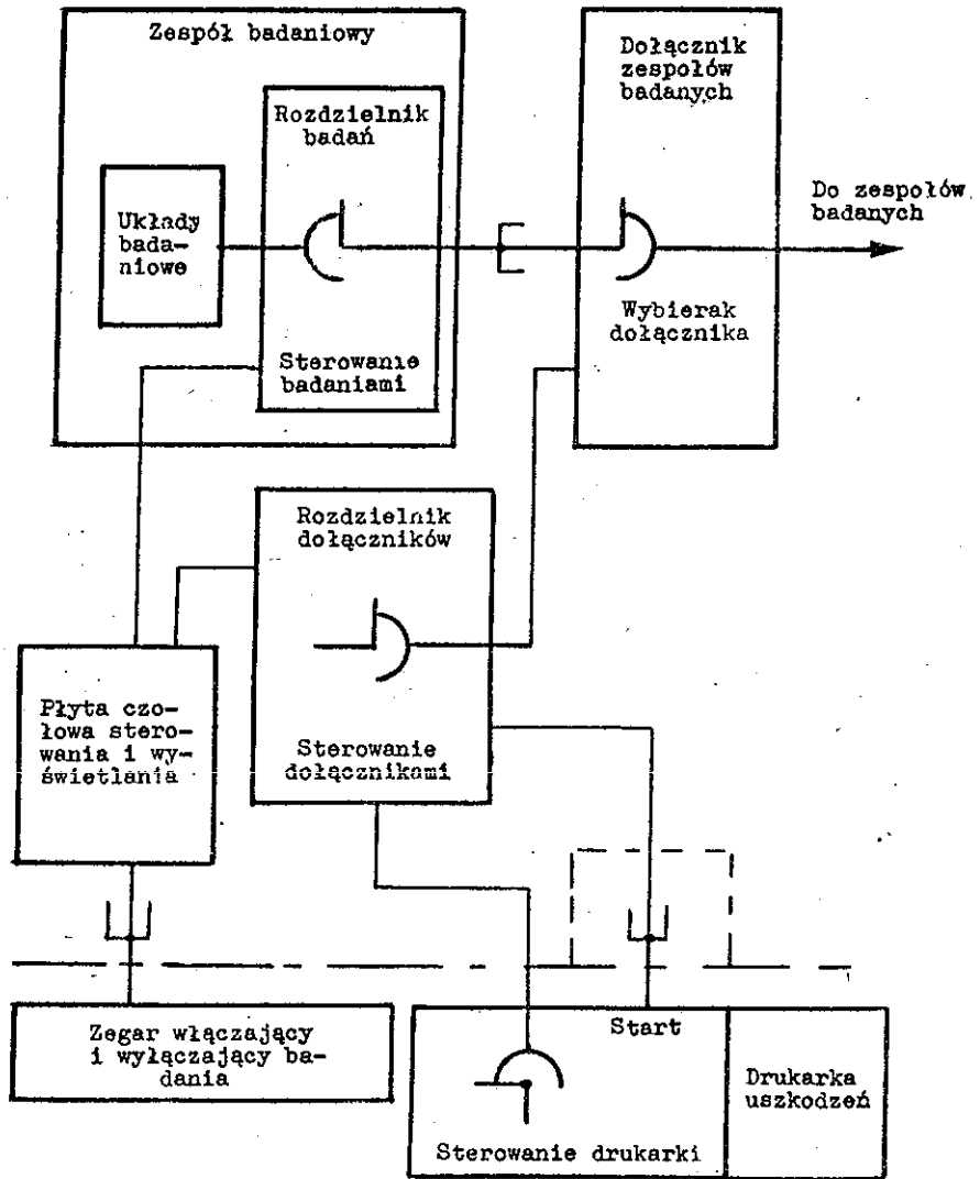
Rys. 16. Ulepszony rutiner
