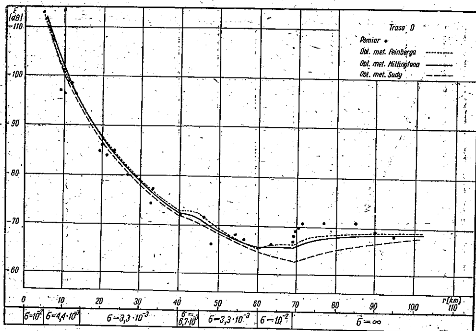
Rys. 13. Wyniki obliczeń rozkładu natężenia pola na trasie D
