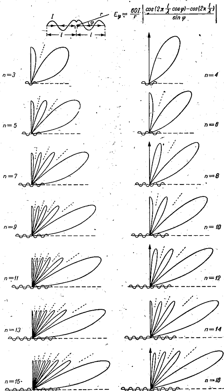
Rys. 5. Charakterystyki wiartkowe promieniowania symetrycznego wibratora prostoliniowego w wolnej przestrzeni
