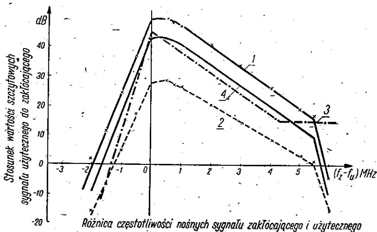
Rys. 4. Krzywe współczynników bezpieczeństwa dla standardu 625 linii i kanału 8 MHz: 1 — krzywa współczynnika bezpieczeństwa dla progu zauważalności interferencji; 2 — krzywa współczynnika bezpieczeństwa dla interferencji uniemożliwiającej obserwację; 3 — krzywa współczynnika bezpieczeństwa z materiałów CCIR (tymczasowa) dla standardu 625 linii; 4 — proponowana krzywa współczynnika bezpieczeństwa dla interferencji dopuszczalnej
