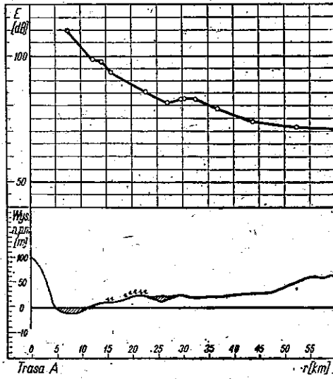
Rys. 5. Trasa A — Profil trasy i wykres natężenia pola
