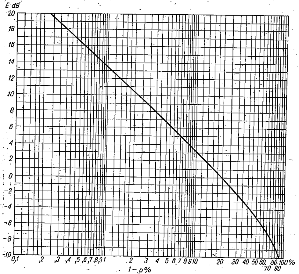
Rys. 3. Natężenie pola E dB ponad wartość E_{0,8} w funkcji prawdopodobieństwa wypadnięcia sygnału 1-p\% (wg S. Manczarskiego)
