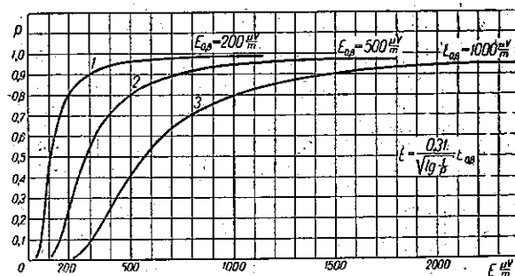
Rys. 2. Współczynnik zrozumiałości p audycji radiofonicznych na falach krótkich ze względu na zaniki jonosferyczne, występujące przy różnych wartościach natężenia pola E fali nośnej, zależnie od poziomu zakłóceń lokalnych (wg S. Manczarskiego);
