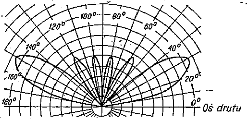
Rys. 6. Charakterystyki połówkowe promieniowania drutu w wolnej przestrzeni (wg W. Jachnowa, Telefunken Mitteilungen, Mai 1940, s. 57)
