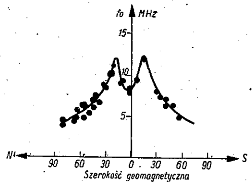
Rys. 18. Zależność częstotliwości krytycznej od szerokości geomagnetycznej (wg Appletona): f_0 — częstotliwość krytyczna przy odbiciu prostopadłym od warstwy F2
