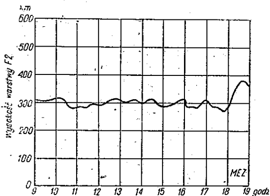
Rys. 14. Zmiany wysokości warstwy F2. (wg pomiarów Eyfriga)
