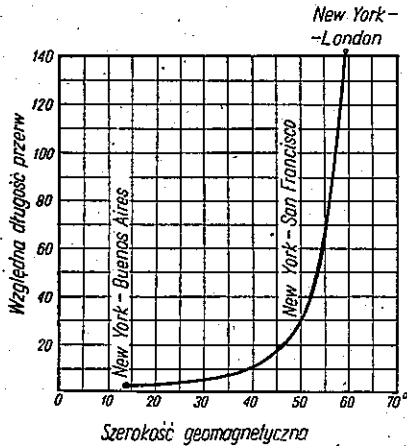
Rys. 19. Względna długość przerw jonosferycznych na różnych trasach w czasie 16 silnych burz magnetycznych (1939—1940): Wg 1) L. V. Berkner and H. W. Wells, Terr. Magn. 42, 183 (1937). Wg 2) M. Waldmeier, Zs. Astroph. 14, 229 (1931). Wg 3) H. E. Halborg, Proc. Amer. Phil. Soc. 84, 323 (1941)
