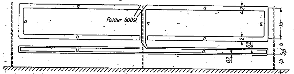
Rys. 9. Schemat dwupoziomowej anteny PBS: a — linka miedziana twarda \phi 4 mm; b — drut stalowy nierdzewny \phi 2,5 mm. Wymiary w metrach. Skala 1:100 (zmodyfikowana przy małych wymiarach)
