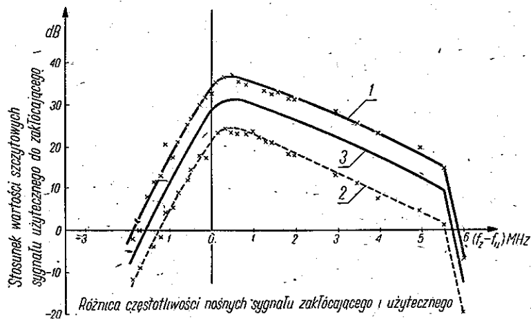
Rys. 5. Krzywe współczynników bezpieczeństwa dla standardu 625 linii i kanału 8 MHz przy odstrojeniach równych pełnej wielokrotności nieparzystej połowy częstotliwości linii: 1 — krzywa współczynnika bezpieczeństwa dla progu zauważalności interferencji; 2 — krzywa współczynnika bezpieczeństwa dla interferencji uniemożliwiającej obserwację; 3 — proponowana krzywa współczynnika bezpieczeństwa dla interferencji dopuszczalnej
