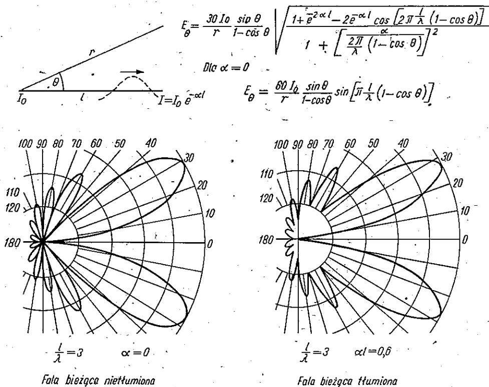
Rys. 7. Charakterystyka promieniowania w wolnej przestrzeni drutu z falą biejącą tłumioną oraz — dla porównania — nietyłmioną
