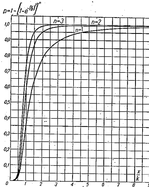
Rys. 1. Prawdopodobieństwo odbioru na falach krótkich przy systemie diversity, składającym się z n anten (wg S. Manczarskiego): x — stosunek wartości skutecznej wygładzonej sygnału do zakłóceń; k — stosunek najsłabszego rozróżnialnego sygnału do zakłóceń
