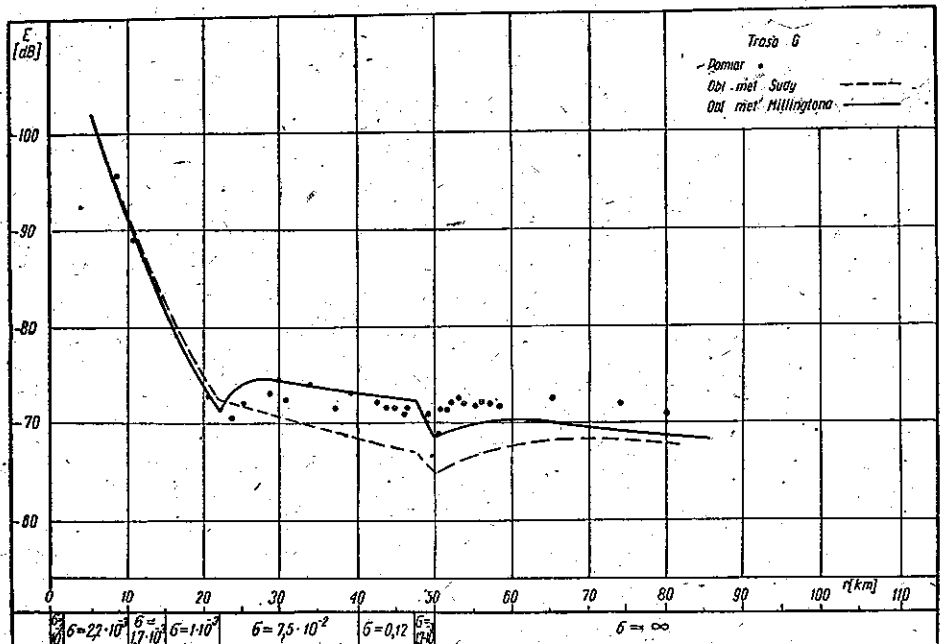
Rys. 15. Wyniki obliczeń rozkładu natężenia pola na trasie G
