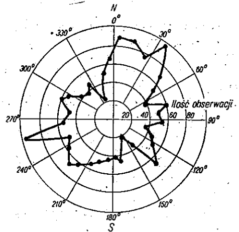
Rys. 12. Rozkład kierunków wiatrów w warstwie F. Niemcy, 1950
