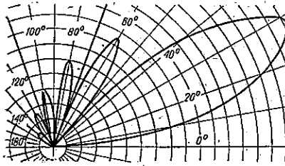
Rys. 6. Charakterystyki połówkowe promieniowania drutu w wolnej przestrzeni (wg W. Jachnowa, Telefunken Mitteilungen, Mai 1940, s. 57)
