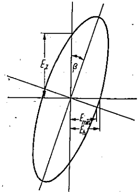
Rys. 3. Elipsa polaryzacji
