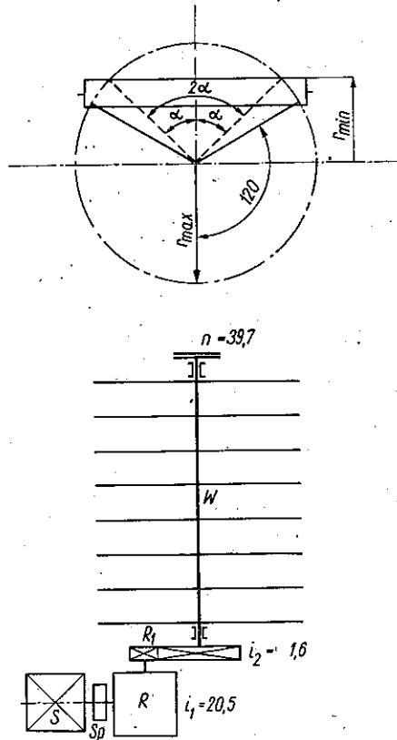
Rys. 4. Układ kinematyczny członu rozdzielczego
