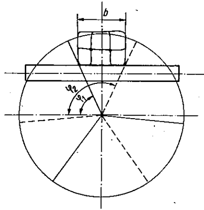
Rys. 12. Położenie ramion zgrniających określone czasem krytycznym
