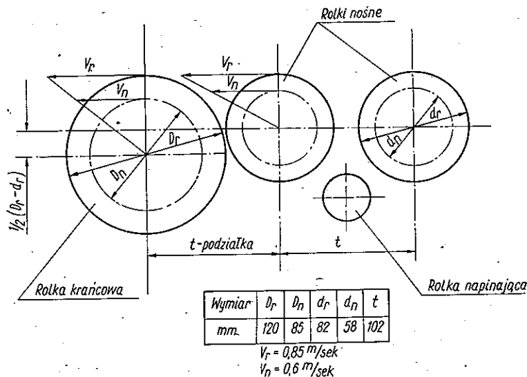
Rys. 3. Schemat napędowy rolek
