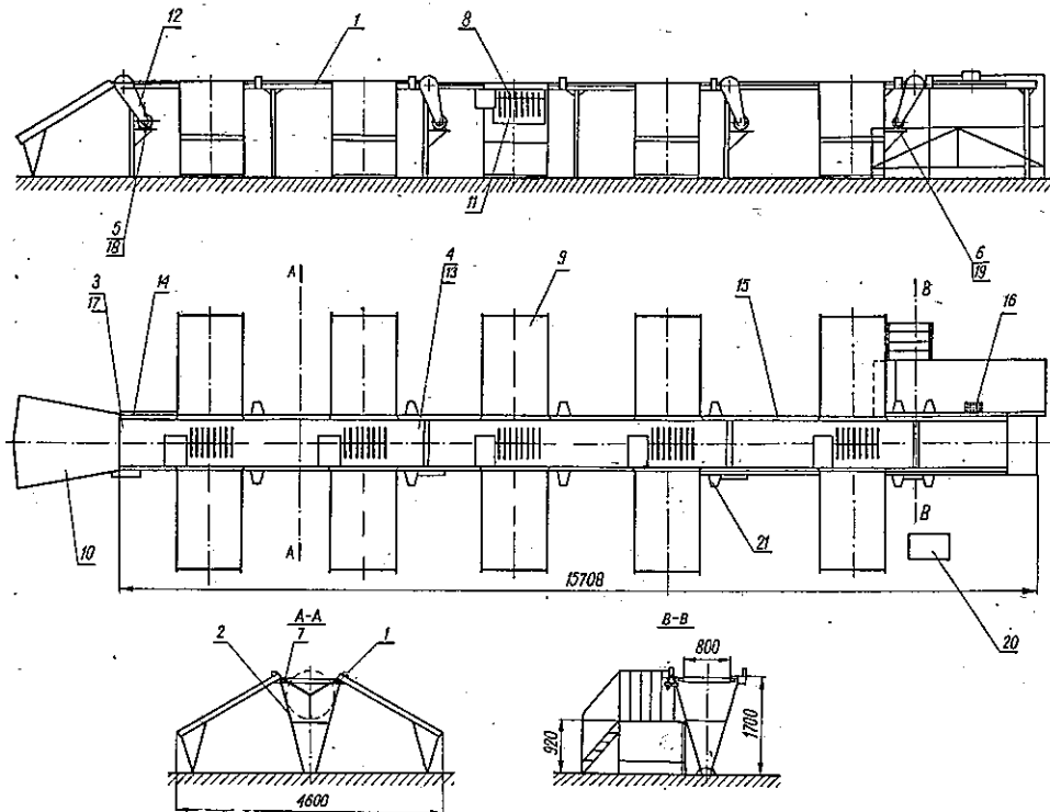
Rys. 2. Schemat konstrukcyjny
