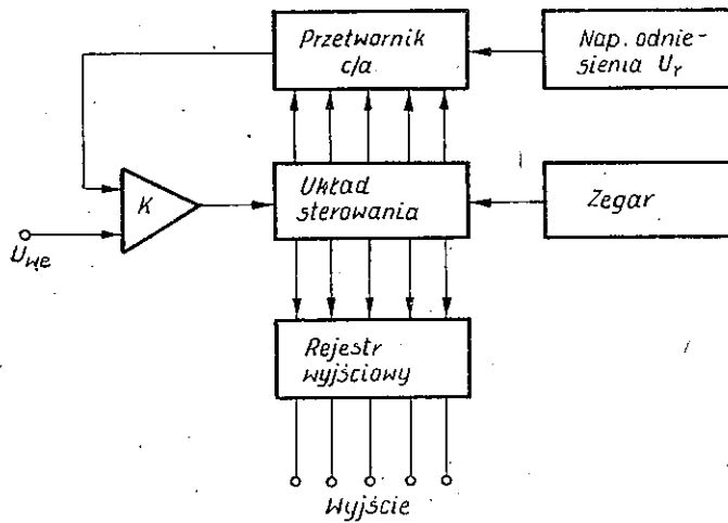
Rys. 3. Schemat blokowy przetwornika a/c z porównywaniem szeregowym
