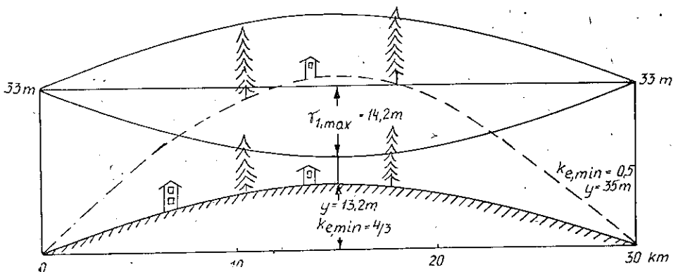
Rys. 13. Warunki propagacji w strefie Fresnela linii 11 GHz o długości 30 km
