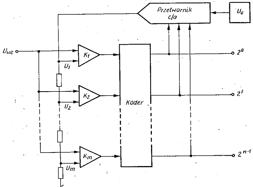
Rys. 4. Schemat blokowy przetwornika a/c szeregowo-równoległego
