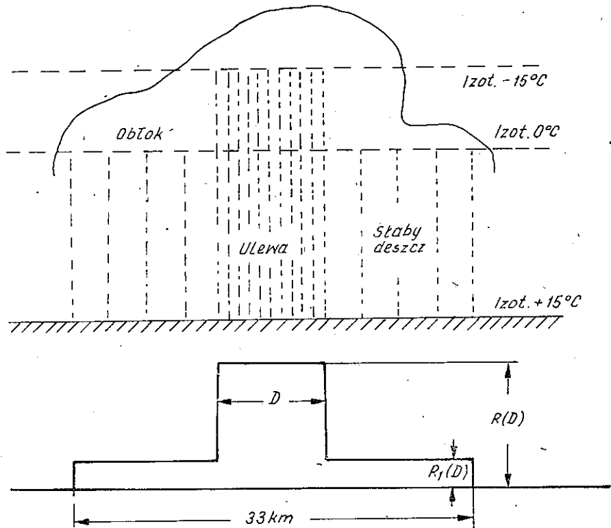
Rys. 4. Model opadu przelotnego
