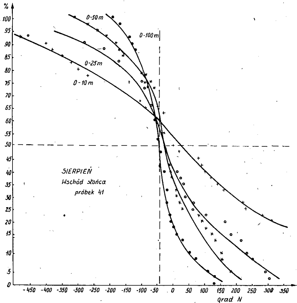
Rys. 1. Rozkłady gradientu wskaźnika refrakcji N w warstwach dla sierpnia o wschodzie słońca
