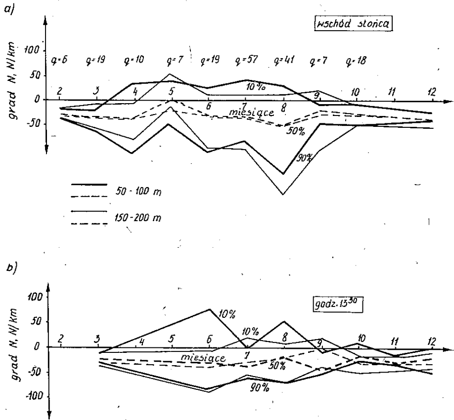
Rys. 10. Roczny cykl decyli 10%, 50% i 90% rozkładów gradientu N a) w warstwach 50-100 m i 150-200 m dla wschodu słońca; b) dla godz. 13.30
