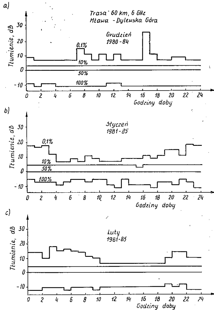
Rys. 7. Dobowy cykl procentu czasu trwania zaników sygnału na trasie Mława - Dylewska Góra dla 0,1%, 10%, 50% i 100% miesiąca a) grudnia, b) stycznia, c) lutego
