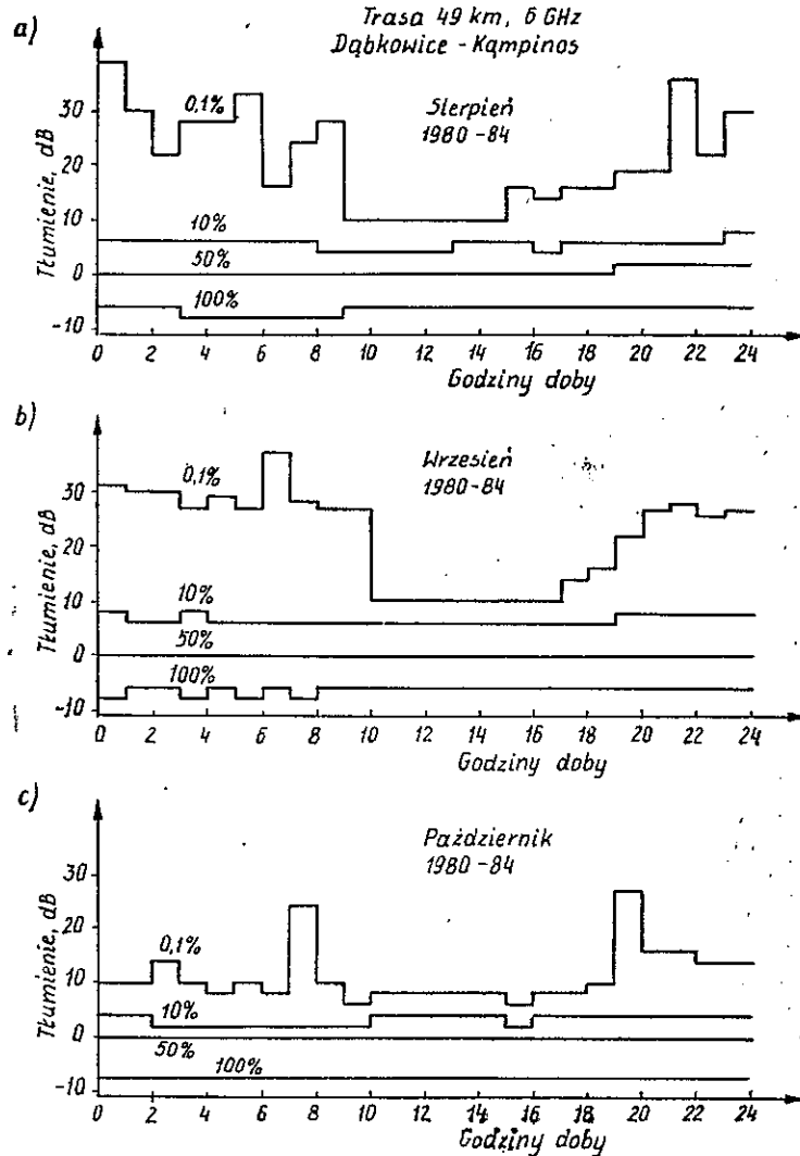
Rys. 9. Dobowy cykl procentu czasu trwania zaników sygnału na trasie Dąbkowice – Kampinos dla 0,1%, 10%, 50% i 100% miesiąca a) sierpnia, b) września, c) października
