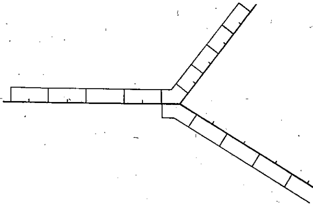
Rys. 2. Szkic wyjaśniający sposób konstrukcji funkcji segmentowych na złączu
