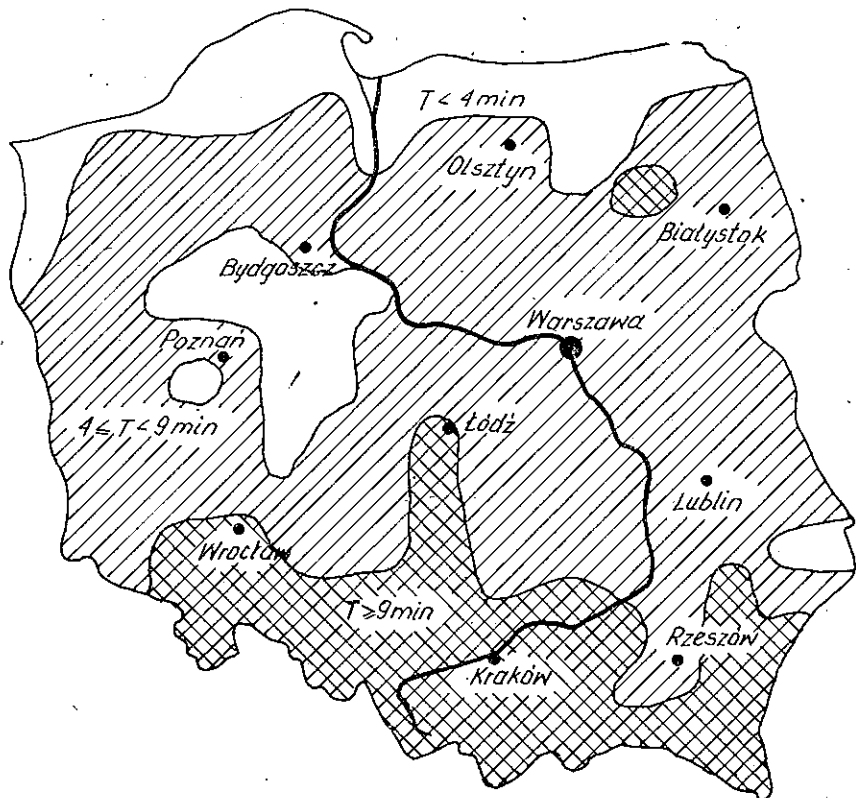
Rys. 1. Czas trwania T minut intensywności opadu R \geq 90 mm/godz. na obszarze Polski w okresie rocznym
