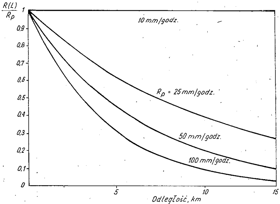
Rys. 5. Model wykładniczy opadu przy \gamma = 0,1
