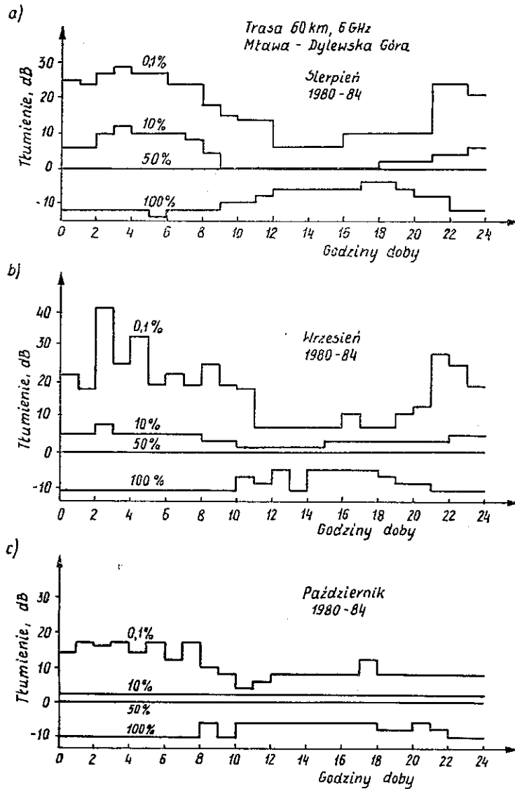
Rys. 6. Dobowy cykl procentu czasu trwania zaników sygnału na trasie Mława – Dylewska Góra dla 0,1%, 10%, 50% i 100% miesiąca a) sierpnia, b) września, c) października
