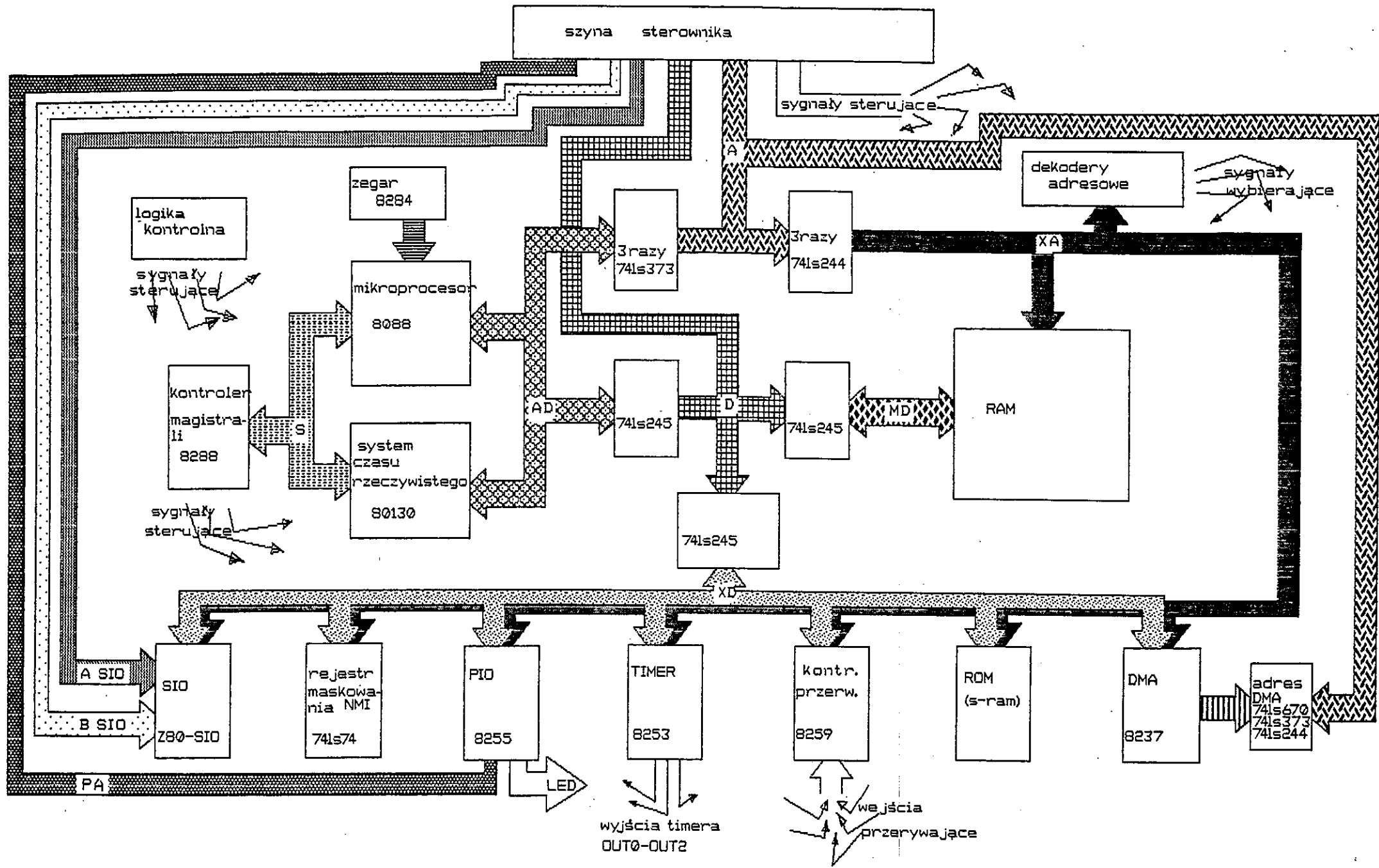
Rys. 1. Schemat blokowy sterownika
