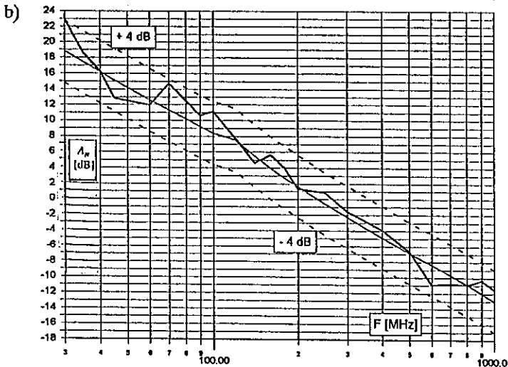
Rys. 4. Zmiany współczynnika A_N w funkcji częstotliwości przy polaryzacji pionowej dla poligonu pomiarowego Instytutu Łączności O/Wrocław przy ul. Swojczyckiej we Wrocławiu
