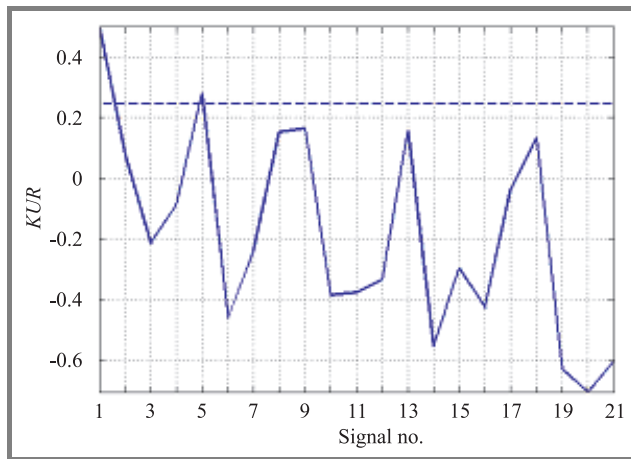
Fig. 4. Kurtosis.
