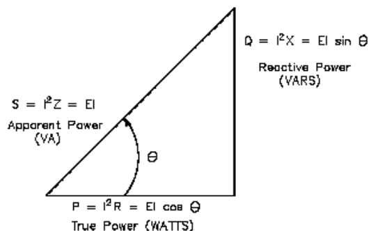
Gambar 1. Segitiga daya
