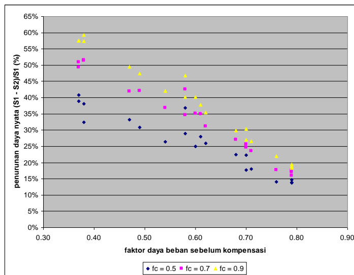
Gambar 3. Penurunan daya nyata instalasi setelah pemasangan kapasitor
