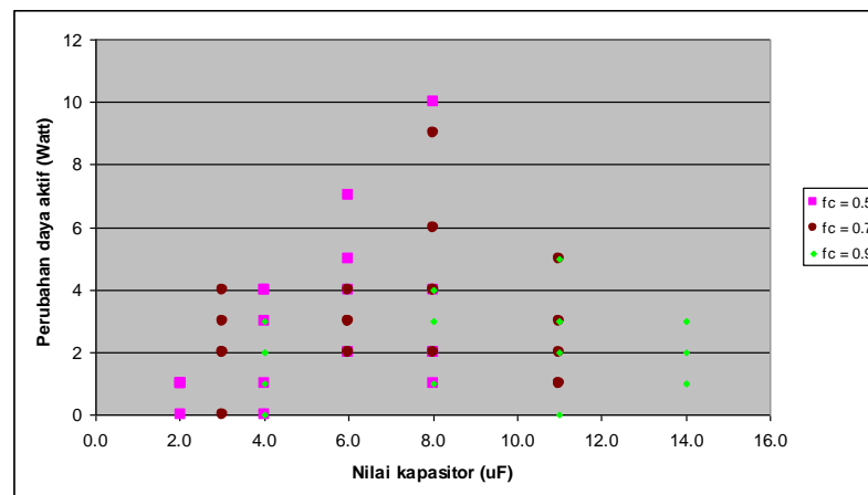
Gambar 5. perubahan daya aktif
