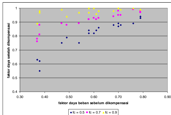
Gambar 4. Perbaikan faktor daya instalasi
