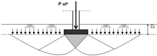
Gambar 1 Skema keruntuhan geser umum pada fondasi dangkal (Terzaghi, 1943)
