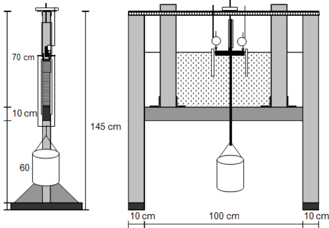
Gambar 5 Skema pengujian dilaboratorium.
