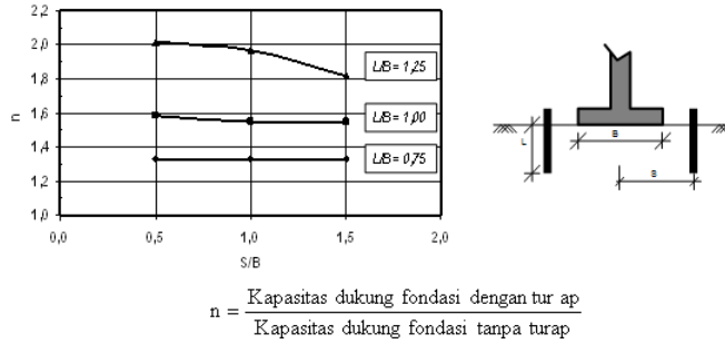
Gambar 8 Hubungan antara letak turap dan kapasitas dukung fondasi dengan turap.
