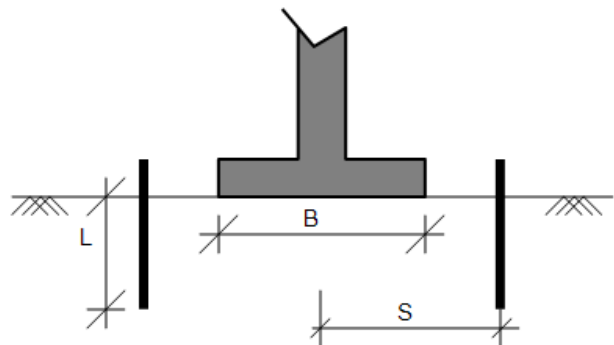
Gambar 4 Skema pemasangan turap pada perkuatan fondasi telapak.
