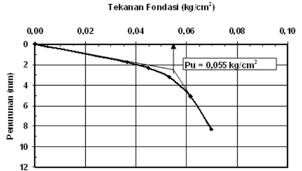
Gambar 6 Hasil pengujian fondasi telapak tanpa tiang.
