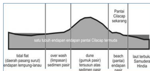
Gambar 1. Satu sekuen tubuh endapan Pantai Cilacap.
