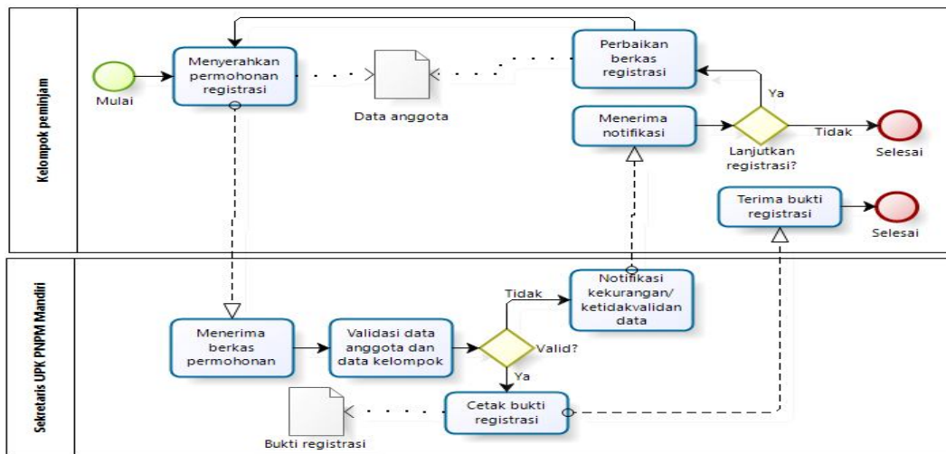
Gambar 7: Diagram proses registrasi peminjam kolektif
