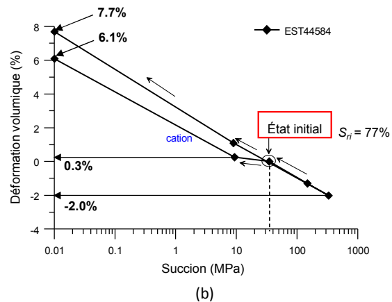
Fig. 2. Propriétés de rétention d'eau de l'argilite du COx (Menaceur 2014) : variation du degré de saturation (a) et de la déformation volumique (b) en fonction de la succion.
