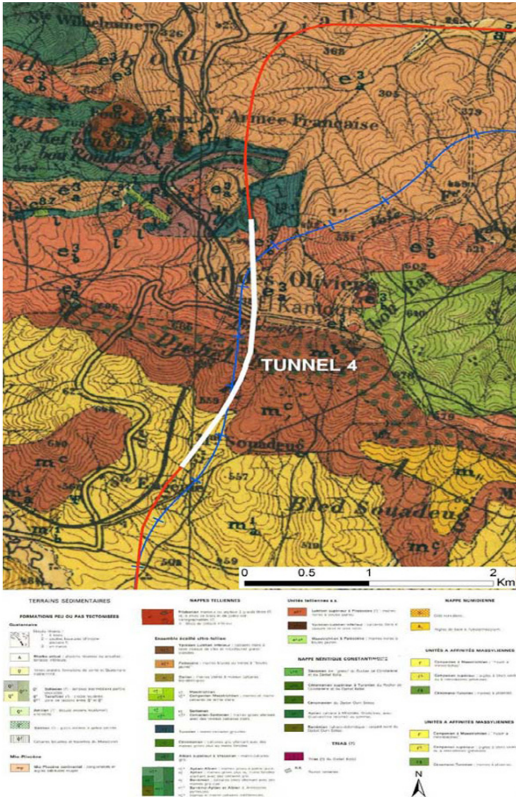
Fig. 2. Tracé du tunnel T4 sur la carte géologique de Smendou.
