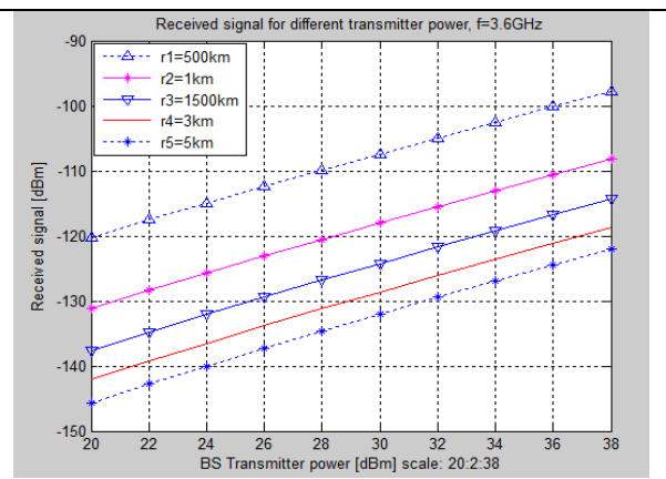
b) F=3.6GHz
