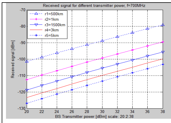
a) F=700MHz
