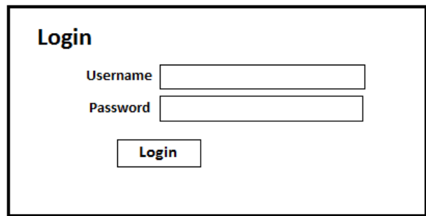
Gambar 10. Halaman Login
