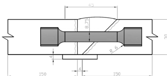
Figura 1 - Esquema de retirada de corpos de prova.
