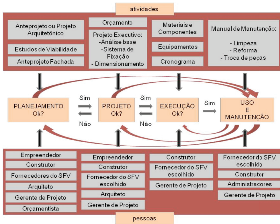
Figura 1: Esquema de especificação do SFV para edificações.
