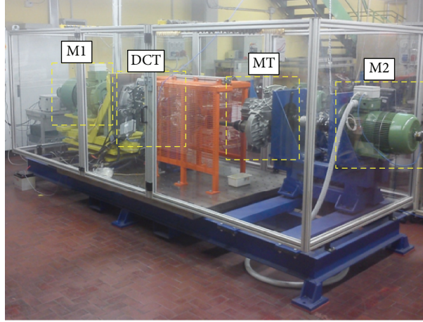
FIGURE 1: Transmission test bench at the Politecnico di Torino.
