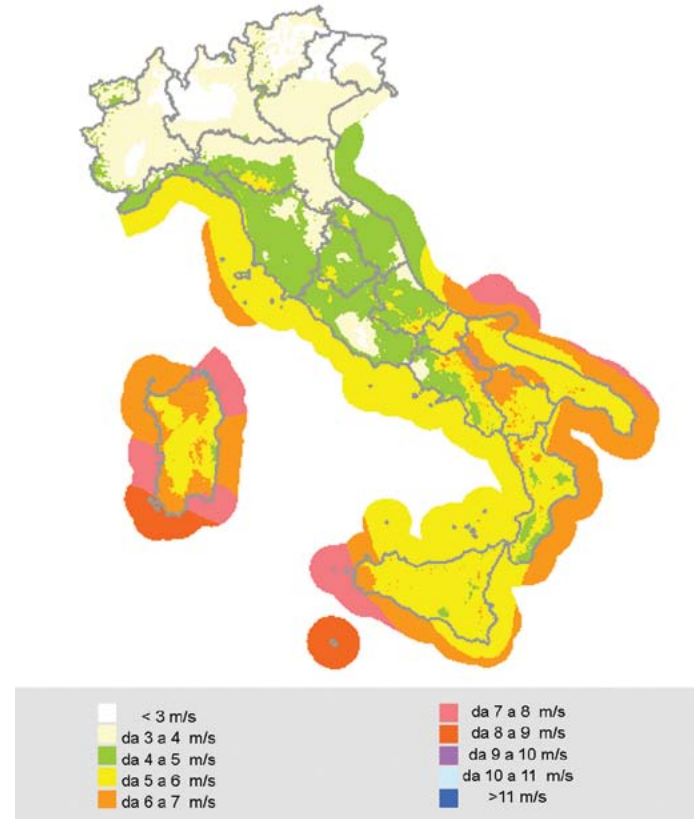
[Fig. 8 - velocità media annua del vento a 50 m s.l.t./s.l.m. - fonte: atlante eolico italiano]
