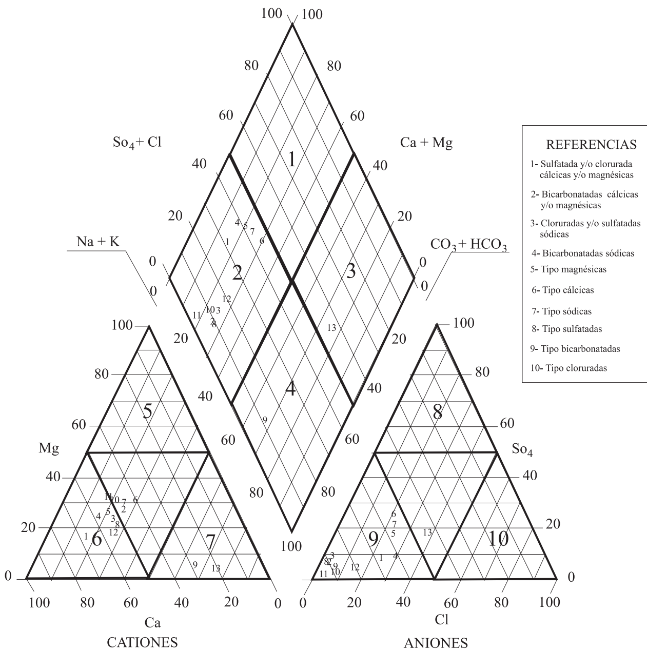
Fig. 2.—Diagrama de representación de los análisis correspondientes a las aguas de los pozos para determinar sus facies químicas.
