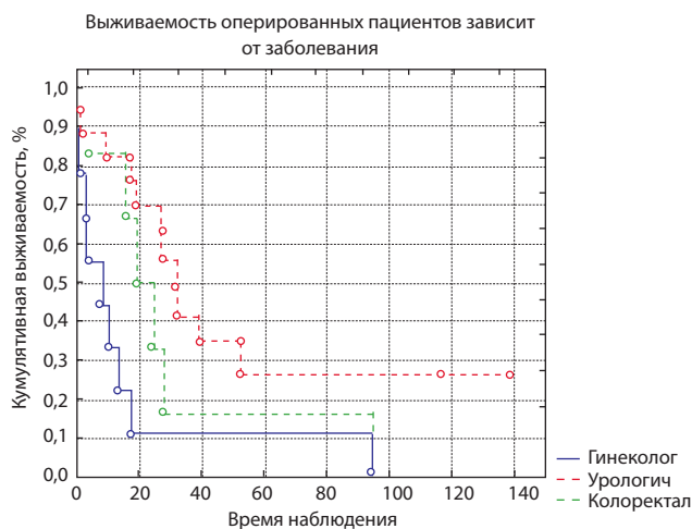
Рис. 5. Выживаемость группы
