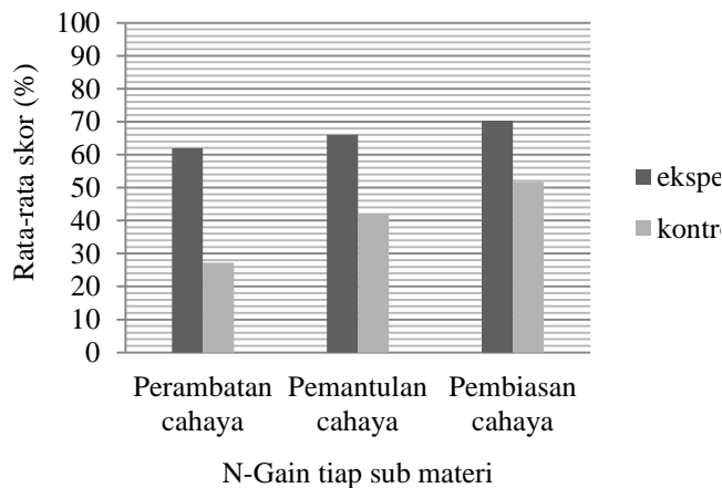
Gambar 2. Nilai Rata-Rata N-Gain Pemahaman Konsep Fisika Siswa Tiap Sub Materi Cahaya Kelas Eksperimen dan Kontrol.
