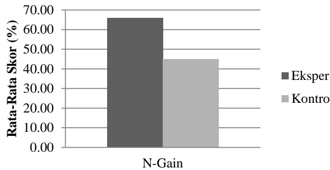
Gambar 1. Nilai Rata-Rata N-Gain Hasil Belajar Fisika Siswa Kelas Eksperimen dan Kontrol
