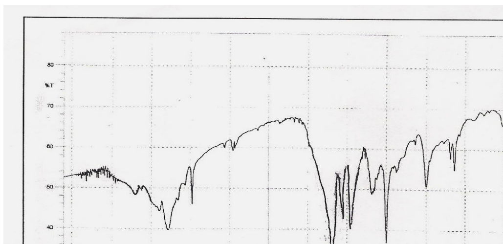
Fig(3) : IR spectrum of \text{NiNO}_2
