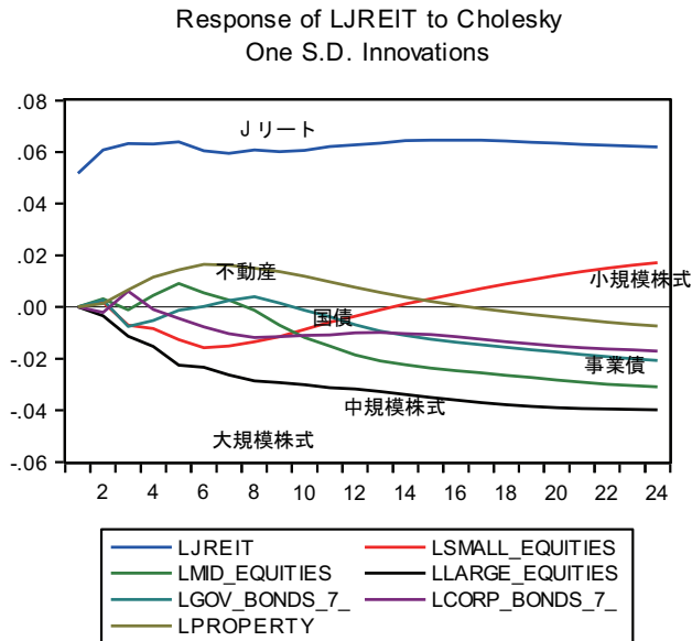
図4.2.4 インパルス応答解析結果（直変化インパルス法、Jリートの応答）
