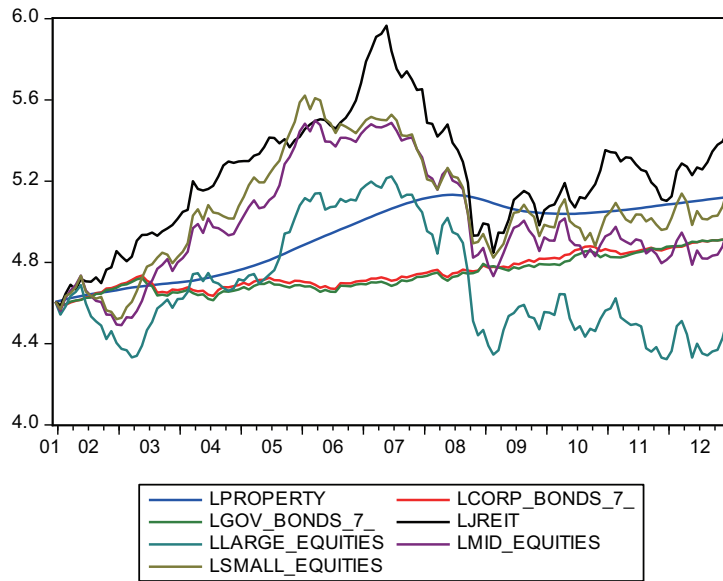
図3.1.2 全指数の推移
