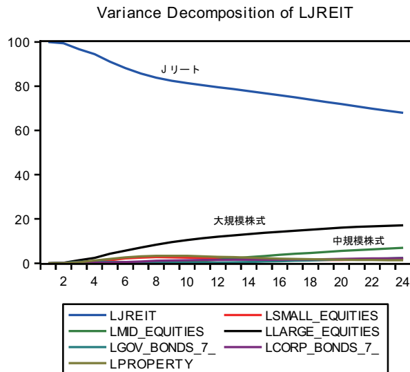
図4.3.4 分散分析（Jリーートの分散分析）
