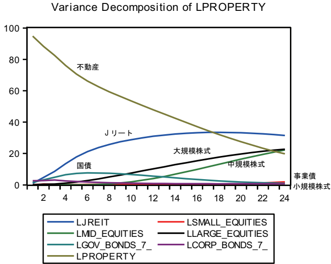
図4.3.3 分散分析（不動産の分散分析）
