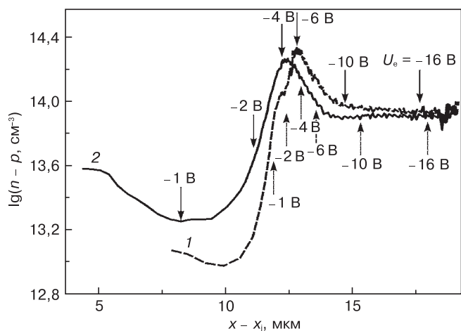
Рис. 4. Профили распределения разности концентраций свободных электронов и дырок, построенные на основе вольт-фарядных характеристик, измеренных при 160 K (1) и 250 K (2). Стрелками указаны границы распространения области пространственного заряда при напряжениях U_e
