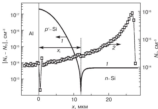
Рис. 1. Расчетные профили: распределения модуля разности концентраций акцепторов и доноров |N_A - N_D| в исходном диоде (1) и распределения первичных вакансий, образованных при облучении диодов ионами криптона с энергией 250 МэВ (2). Флюенс облучения \Phi = 10^8 \text{ см}^{-2}
