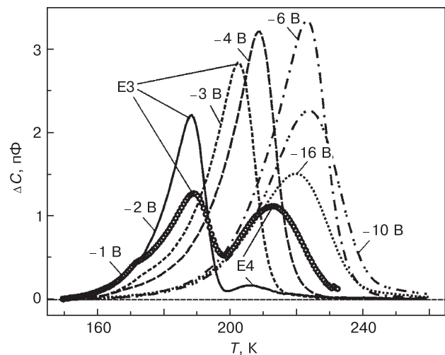
Рис. 3. Спектры DLTS диодов, облученных ионами криптона с энергией 250 МэВ. Флюенс облучения \Phi = 10^8 \text{ см}^{-2} . Длительность импульса заполнения ловушек t_p = 10 \text{ мс} , длительность импульса регистрации релаксации емкости (импульса эмиссии) t_e = 15 \text{ мс} . Напряжение заполнения ловушек U_p = 0 . Значения U_e указаны на рисунке
