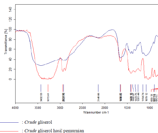
Gambar 2. Spektra IR Crude Gliserol dan Crude Gliserol Hasil Pemurnian
