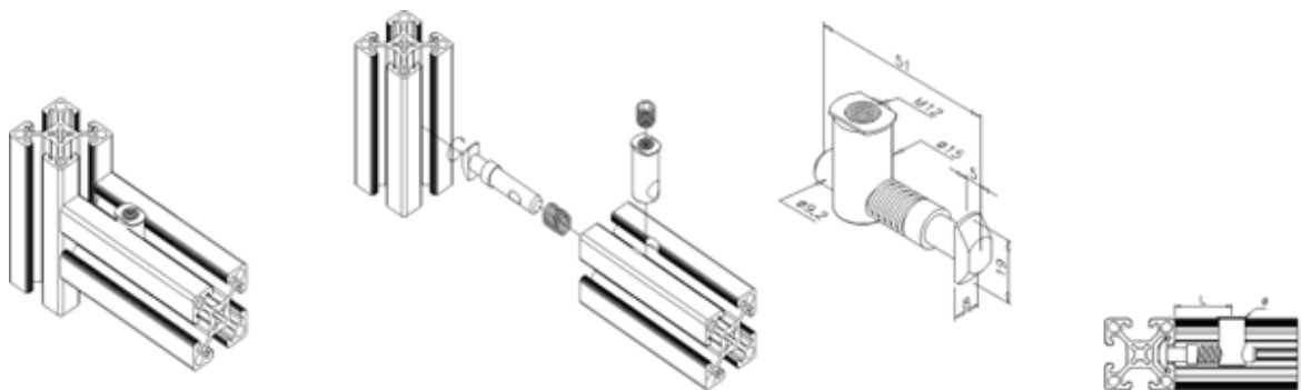
Figura 3.8. Conector de Perfiles Perpendicular
