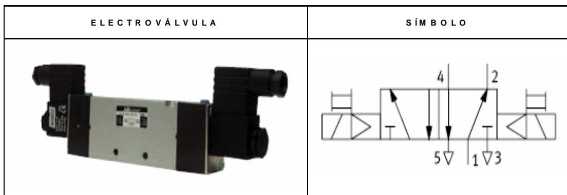
Figura 2.6. Electroválvula 5/2 Biestable 24V.
