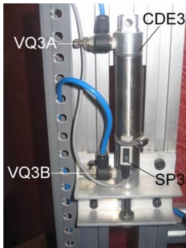
Figura 3.20. Elementos Neumáticos en Módulo de Verificación.
