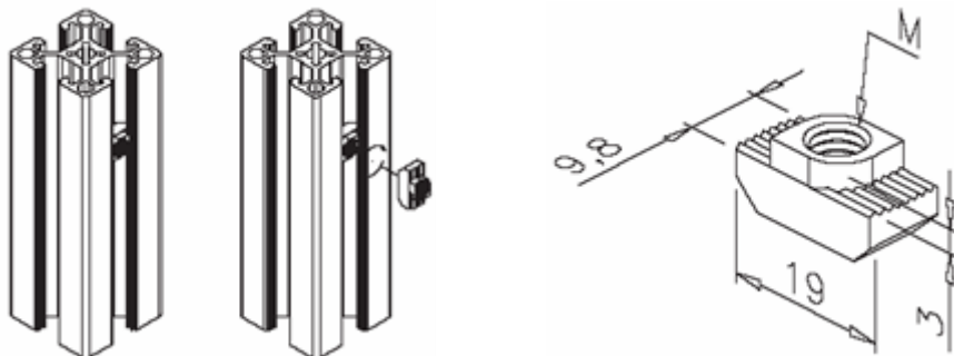
Figura 3.9. Tuerca Cabeza de Martillo.
