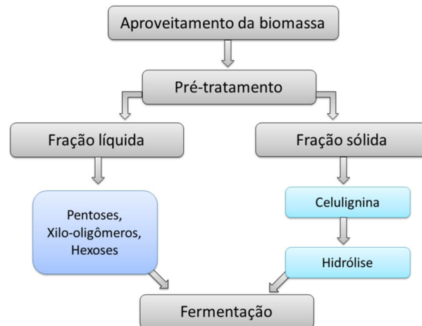
Figura 1 - Esquema dos processos pós a etapa de pré-tratamento da biomassa
