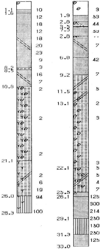
図 7 FAX 出力のボーリング柱状図 Fig. 7 Columnar picture of boring data by FAX
