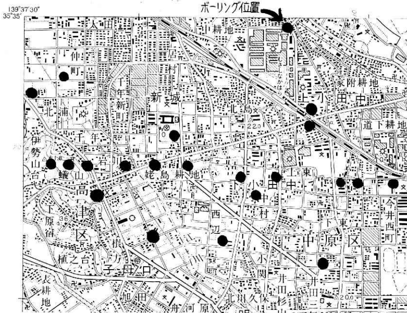
図 4 ボーリング位置をプロットした地形図 Fig. 4 Topographical map plotting the boring location
