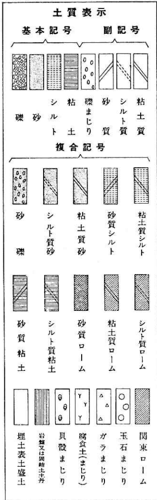
図 6 柱状図の CRT 出力パターン Fig. 6 Output pattern of columnar picture on C.R.T.
