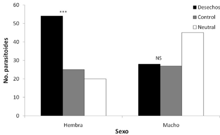
Figura 3. Respuesta de hembras y machos de Prorops nasuta mostrada a los desechos alimenticios y fecales (DAF) o el control. El * indica diferencia significativa ( P < 0.05 ), NS indica diferencia no significativa ( P > 0.05 ). Las hembras que no respondieron a los olores provenientes de los desechos o al control fueron consideradas neutrales.
