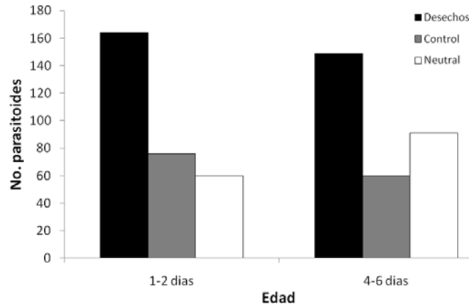
Figura 2. Interacción entre la edad (1-2 días y 4-6 días) y tipo de respuesta (desechos, control, neutral) en hembras de Prorops nasuta . DAF, desechos alimenticios y fecales. Las hembras que no respondieron a los olores provenientes de los desechos o al control fueron consideradas neutrales.
