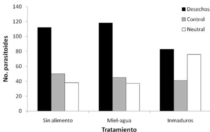
Figura 1. Interacción entre el tipo de alimento (miel-agua, inmaduros y sin alimento) y el tipo de respuesta (desechos, control, neutral) de hembras de Porops nasuta . DAF, desechos alimenticios y fecales. Las hembras que no respondieron a los olores provenientes de los desechos o al control fueron consideradas neutrales.
