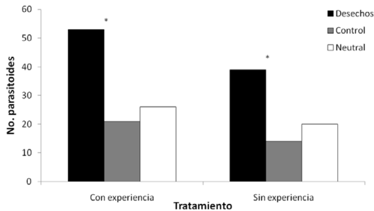
Figura 4. Respuesta de Prorops nasuta con y sin experiencia en oviposición a los desechos alimenticios y fecales (DAF) o el control. * indica diferencia significativa ( P < 0.05 ). Las hembras que no respondieron a los desechos olores provenientes de los o al control fueron consideradas neutrales.
