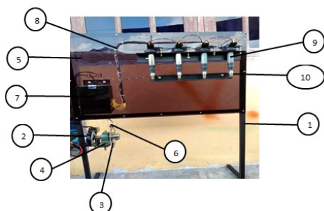
Gambar 2. Alat Simulasi Sistem Pengapian Mesin Bensin 4 Langkah (4 silinder) Berbasis mikrokontroler Arduino Uno.
