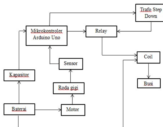
Gambar 3. Diagram Alur Sistem Pengapian
