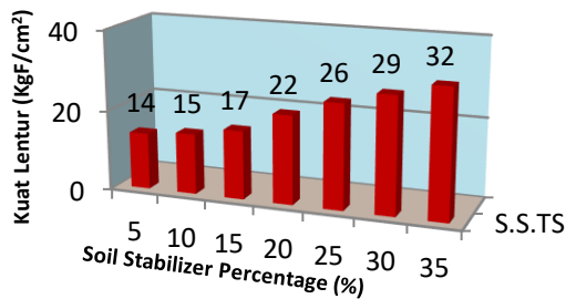
Gambar 4. Hubungan % soil stabilizer dengan kuat lentur sampel.
