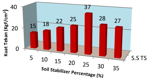
Gambar 5. Hubungan % soil stabilizer dengan kuat tekan sampel.
