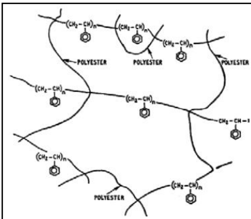
Gambar 2. Struktur polyester jenuh sesudah waktu curing menggunakan inisiator MEKP..
