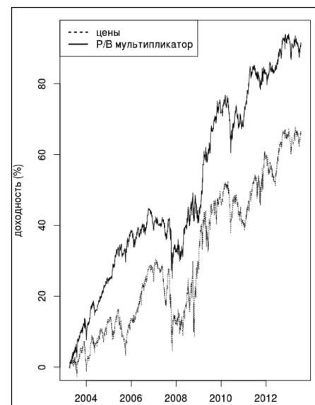
Рис. 1. Кривые капитала арбитражных стратегий в секторе Oil & Gas Production
