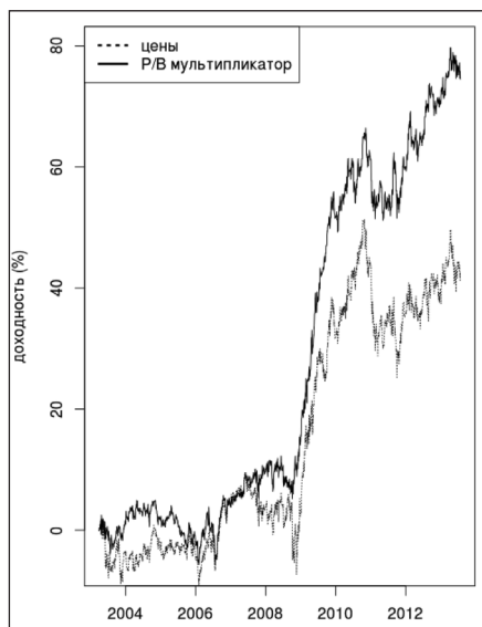
Рис. 2. Кривые капитала арбитражных стратегий в секторе Semiconductors
