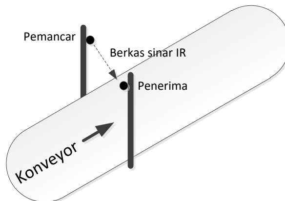
Gambar 3 Rancangan sensor
