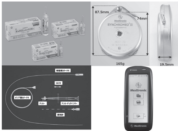
図 2 ITB療法に使用する薬剤および物品 ギャバロン ® 髄注（左上）、シンクロメッド II ® ポンプ（右上）、アシスポンジ ® （左下）、アシスチューブ ® （左下）、エスピジョン ® （右下）
