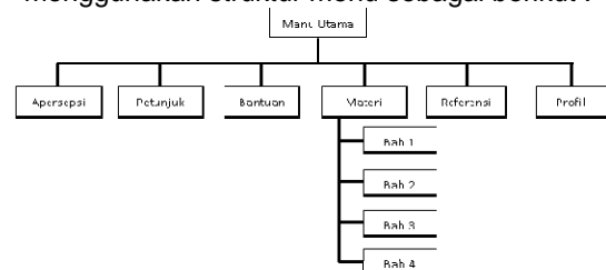
Gambar 2. Struktur Menu
