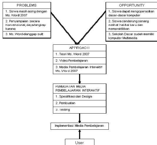
Gambar 1. Kerangka Pemikiran
