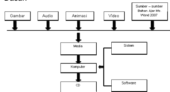
Gambar 4. Kerangka Program
