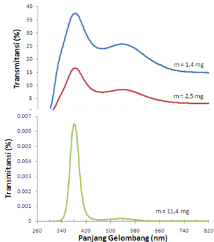
Gambar 3. Pola nilai transmitansi optik untuk nanolayer dengan massa sumber yang berbeda.
