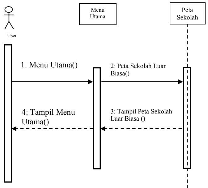
Gambar 6 Sequence Diagram Peta Sekolah Luar Biasa
