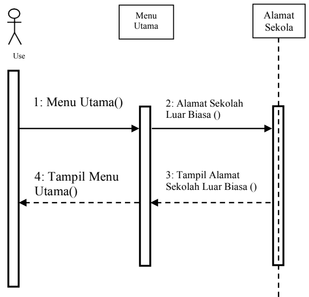
Gambar 5 Sequence Diagram Alamat Sekolah Luar Biasa
