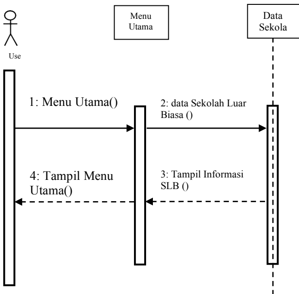
Gambar 4 Sequence Diagram data Informasi Sekolah Luar Biasa
