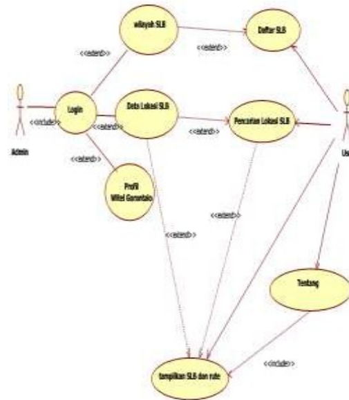
Gambar 1. Use Case Diagram Sistem Yang Diusulkan
