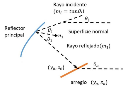
Figura 7. Reflector parabólico con offset array-feed .
