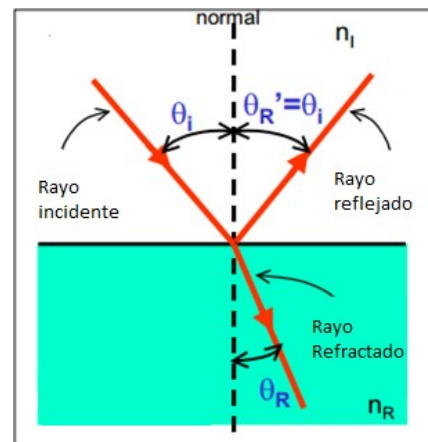
Figura 2. Refracción
