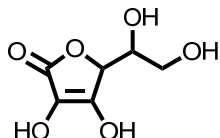
図2 ビタミンC (L-アスコルビン酸)
