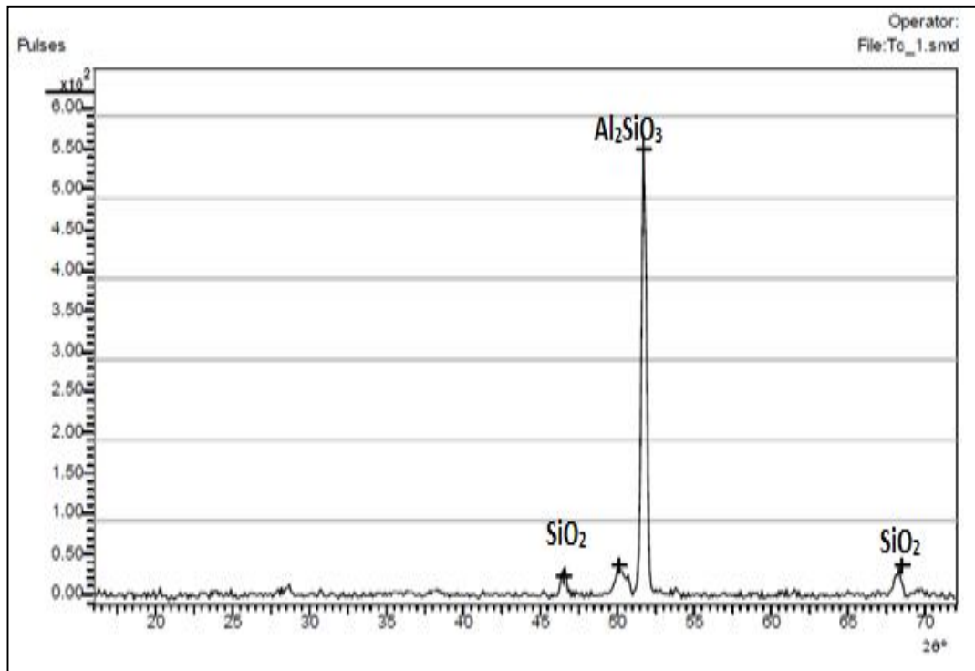
Plate 3 : XRD spectrum for Feldspar
