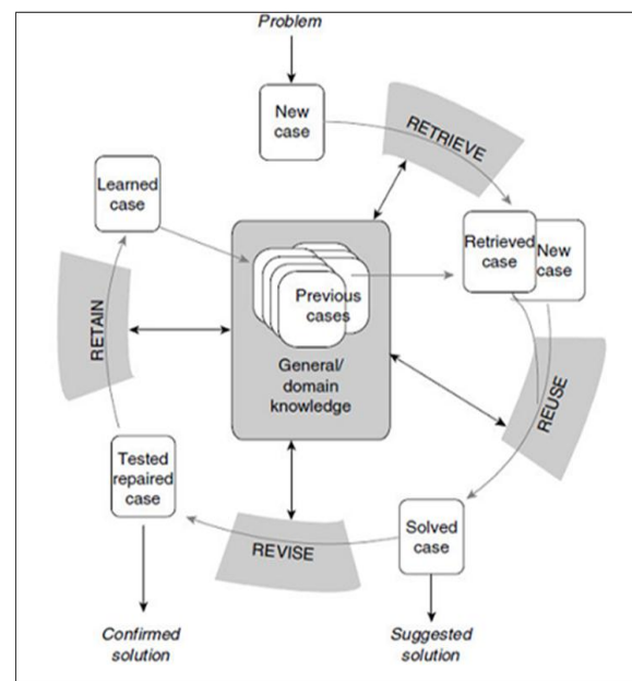
Gambar 1. Siklus CBR
