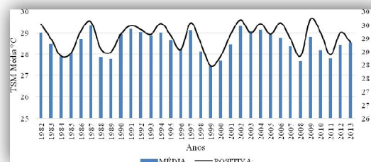
Gráfico 3: Evolução da temperatura da superfície do mar de (1982-2013) Niño 4.
