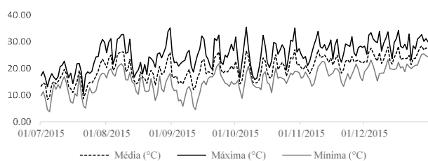
Figura 1 - Médias de temperatura, no local (29°09'S e 56°33' W) e período de realização do experimento.
