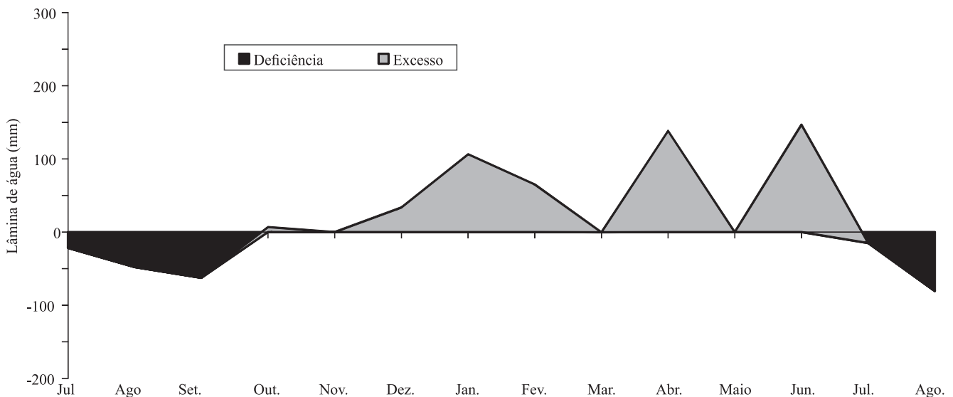
Figura 2. Balanço hídrico mensal, durante o período de julho de 2011 a agosto de 2012.
